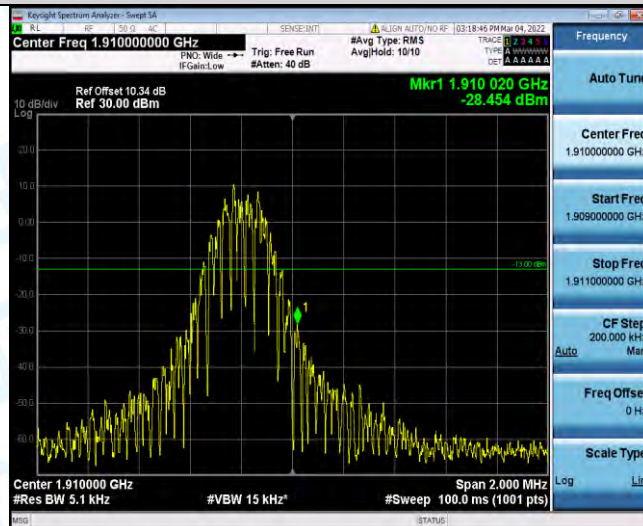
EGPRS1900-810-2
