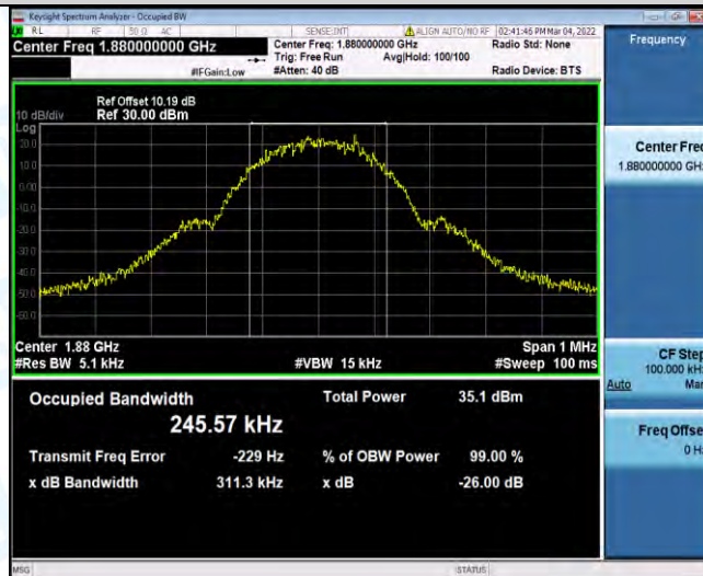
GSM1900-810-0-0.3113
