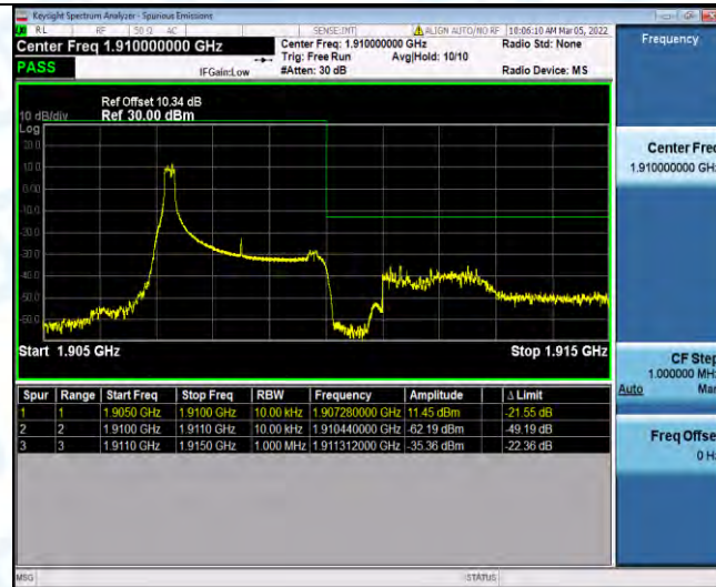
Band2-3MHz-QPSK-19185-1RB#14
