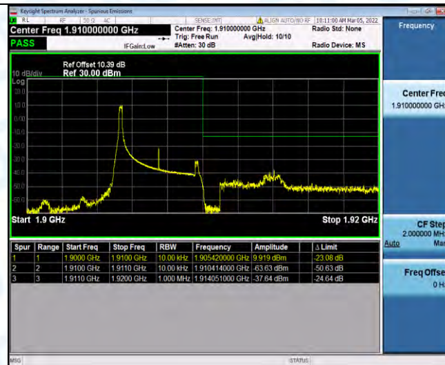
Band2-5MHz-QPSK-19175-1RB#24
