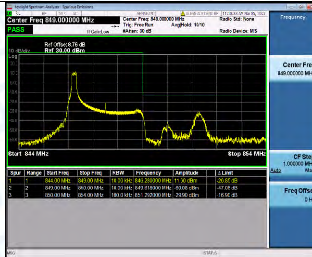
Band5-3MHz-QPSK-20635-1RB#14
