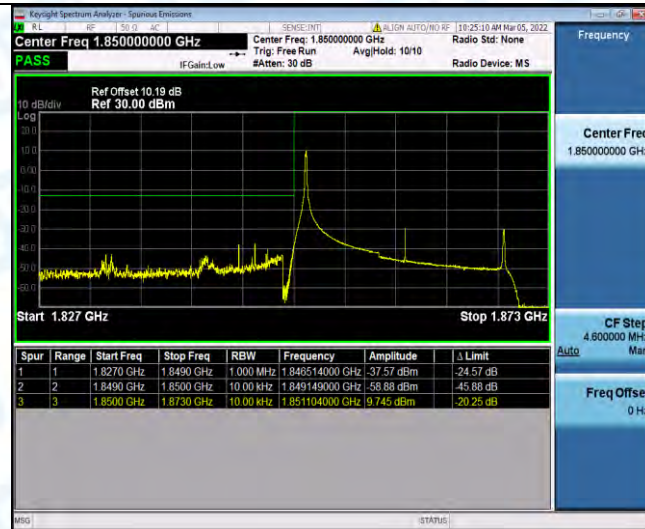
Band2-20MHz-QPSK-18700-1RB#99
