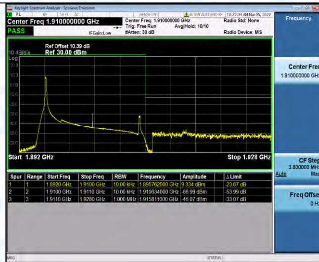
Band2-15MHz-16QAM-19125-1RB#74
