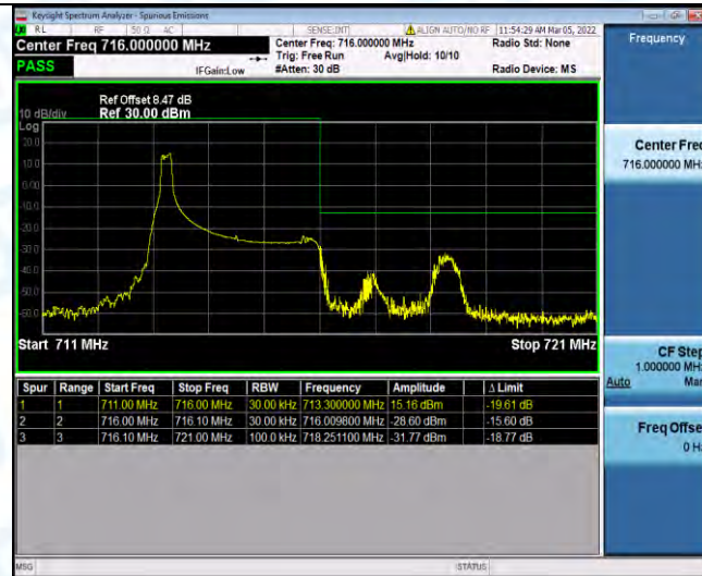
Band12-3MHz-QPSK-23165-1RB#14
