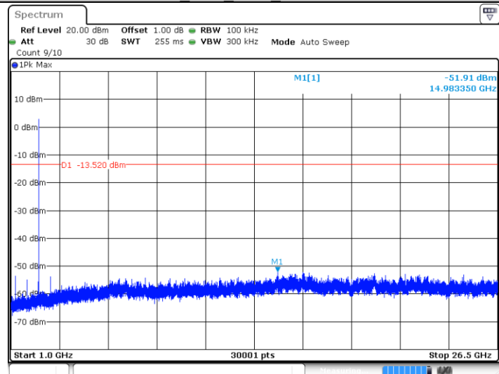
3DH5 Ant1 2441 1000~26500
