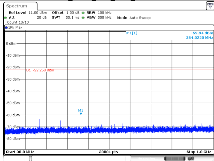
BLE BT4.0 Ant1_2402_30~1000
