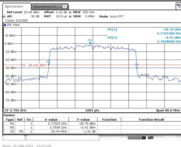
11AX40MIMO_Ant2_5795 484/65
