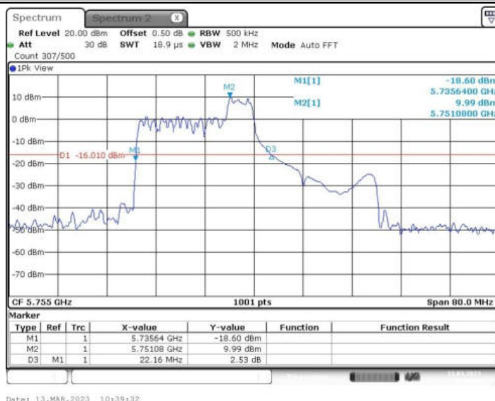
11AX40MIMO_Ant2_5755 52/40
