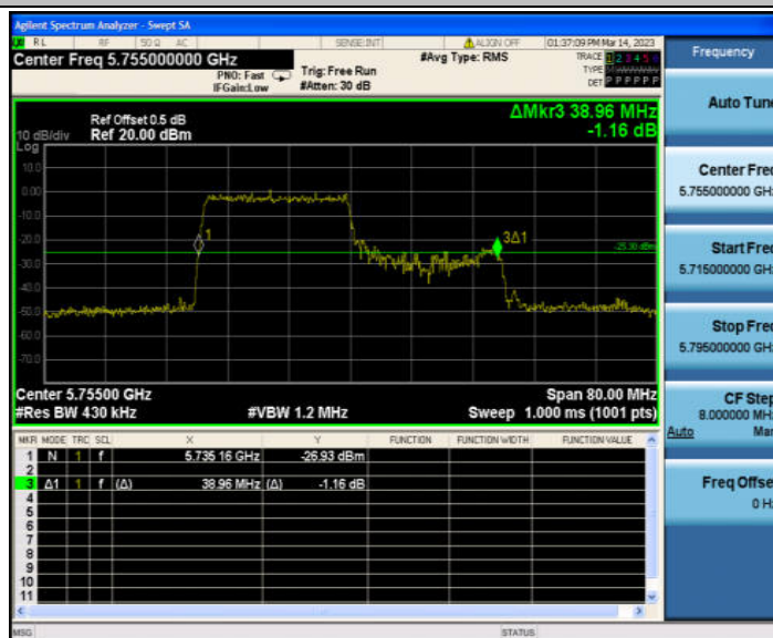
11AX40MIMO_Ant1_5755 484/65
