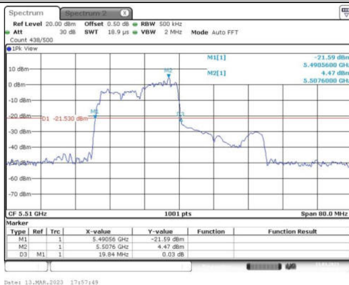
11AX40MIMO_Ant2_5510 106/54
