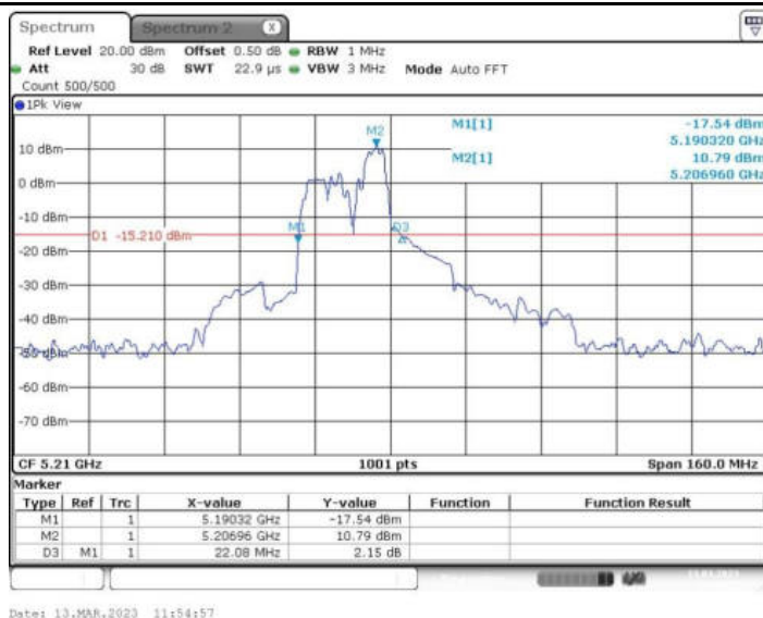
11AX80MIMO_Ant1_5210 106/54
