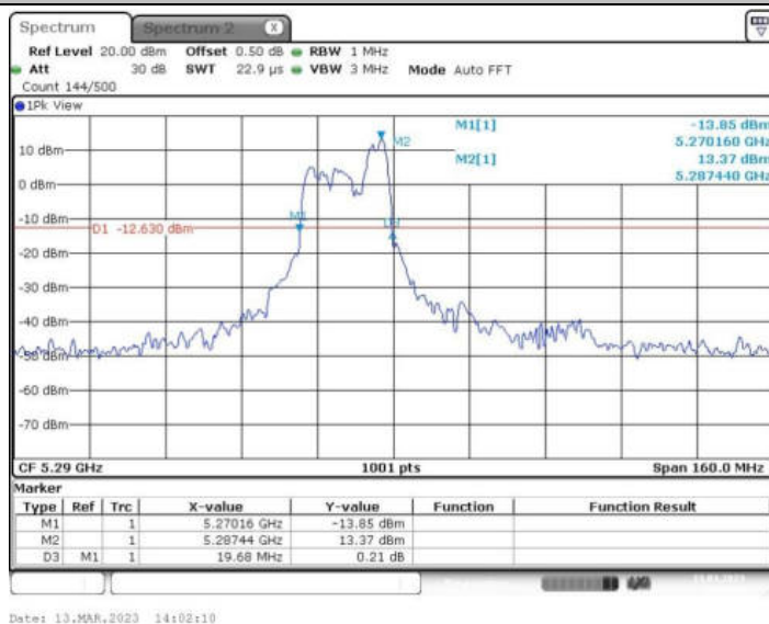
11AX80MIMO_Ant2_5290 52/44
