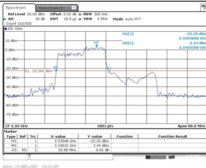
11AX40MIMO_Ant2_5550 106/54
