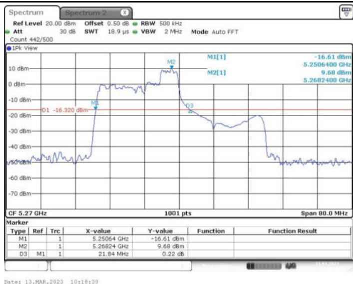
11AX40MIMO_Ant1_5270 106/54
