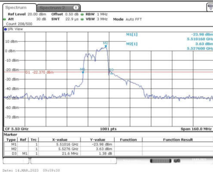
11AX80MIMO_Ant1_5530 242/62
