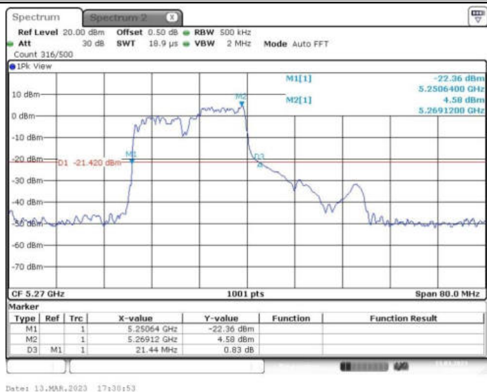
11AX40MIMO_Ant2_5270 106/54
