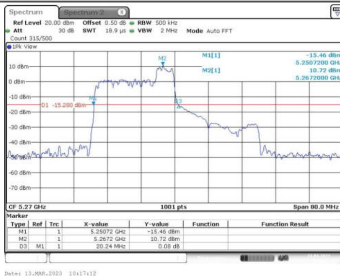
11AX40MIMO_Ant2_5270 52/40
