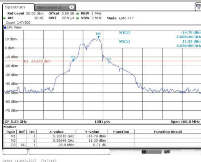
11AX80MIMO_Ant2_5530 106/54
