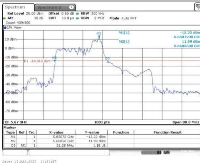
11AX40MIMO_Ant2_5670 52/40
