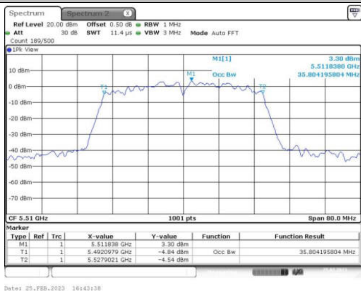
11AC40MIMO_Ant2_5510
