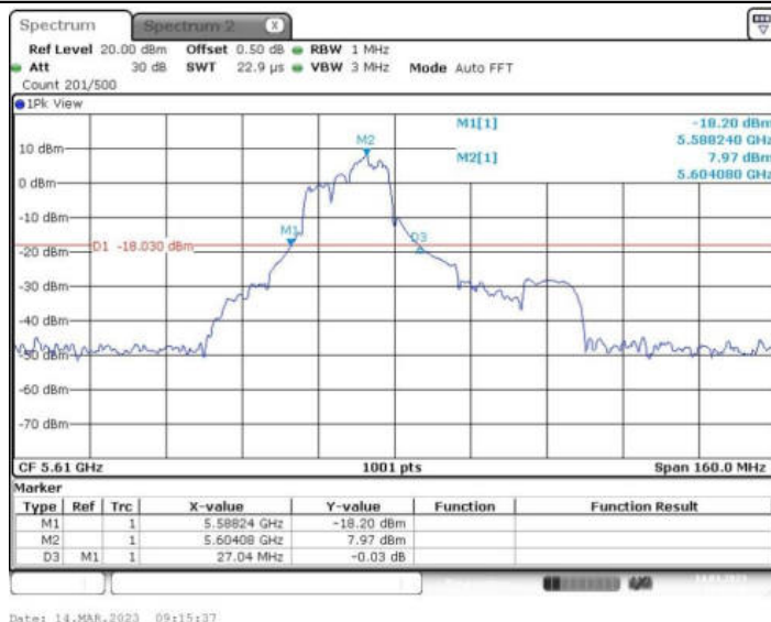
11AX80MIMO_Ant1_5610 242/62
