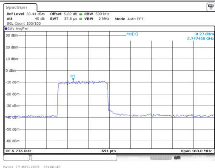
11AX80MIMO_Ant1_5775 996/67
