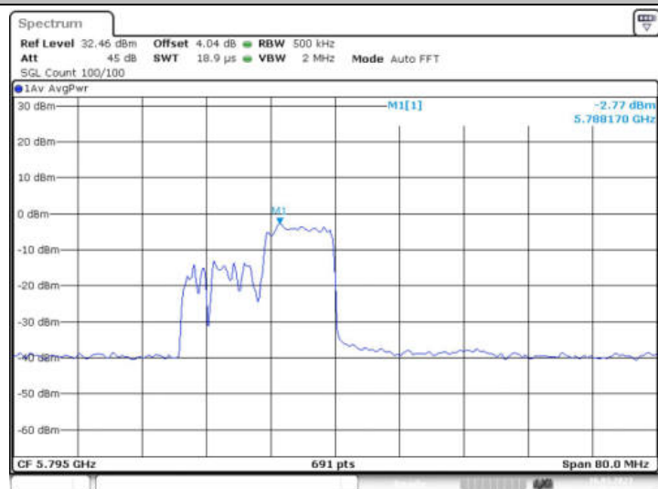
11AX40MIMO_Ant2_5795 106/54
