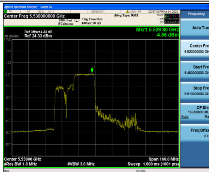
11AX80MIMO_Ant1_5530 484/65
