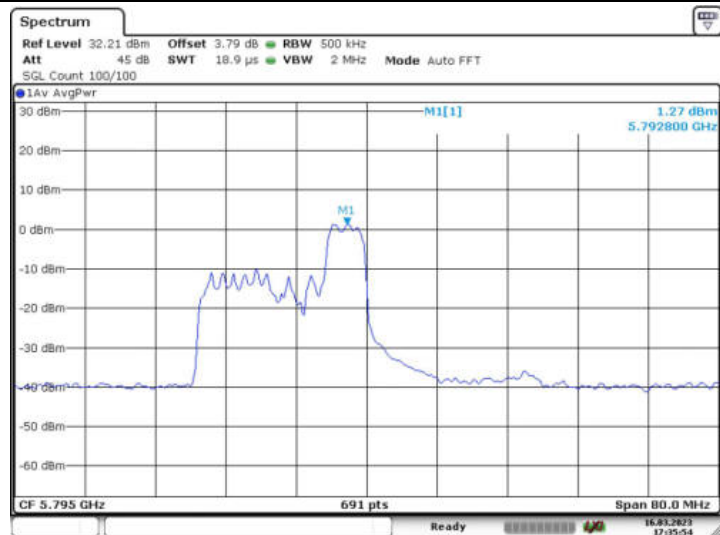
11AX40MIMO_Ant1_5795 106/54
