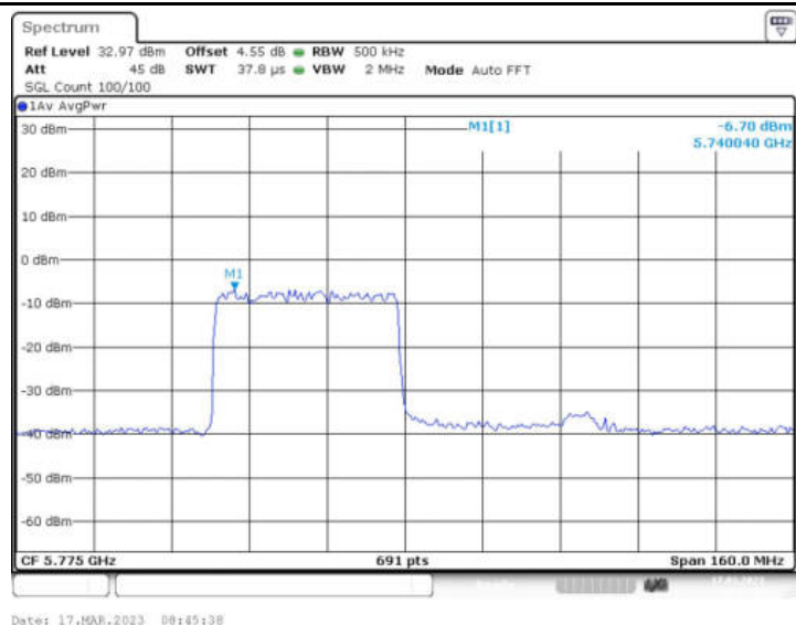
11AX80MIMO_Ant2_5775 484/65
