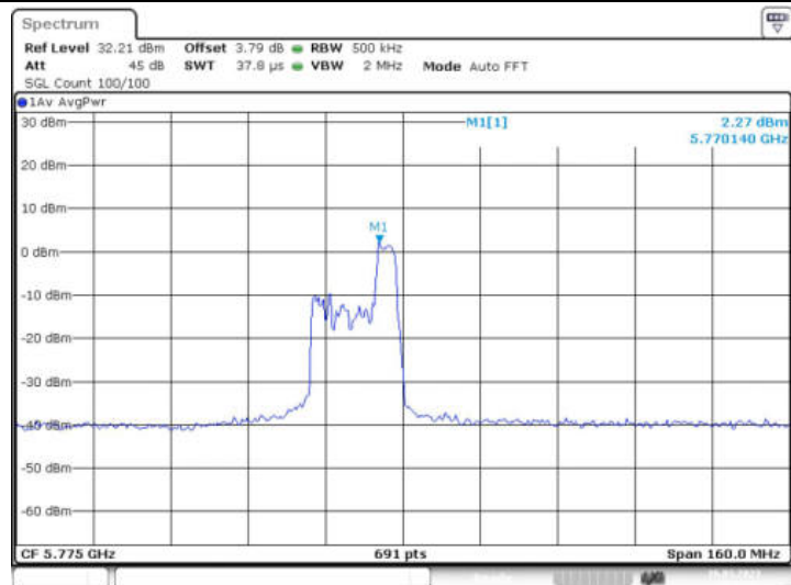
11AX80MIMO_Ant1_5775 106/56
