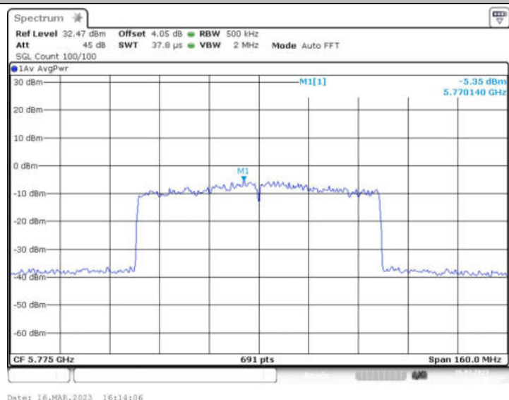
11AX80MIMO_Ant1_5775 996/67
