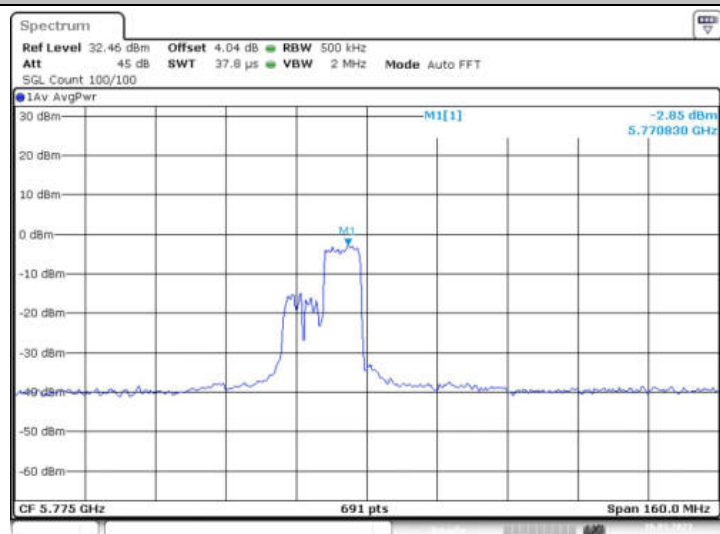
11AX80MIMO_Ant2_5775 106/56
