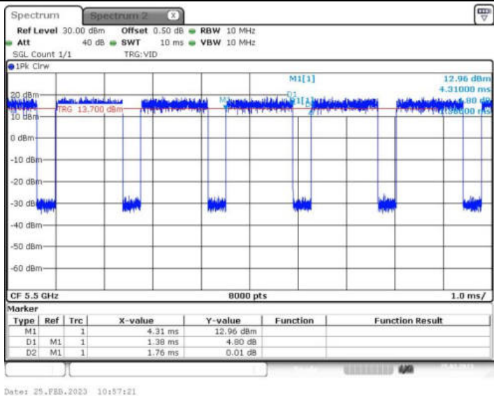
11A_Ant2_5500
