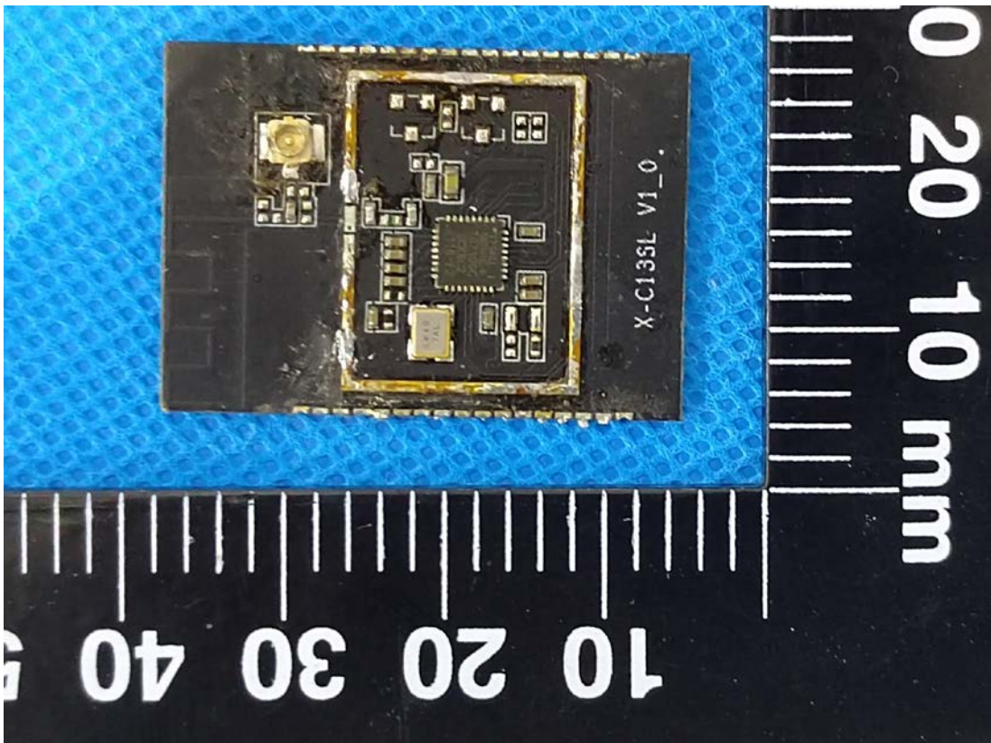
X-C13SL-0
