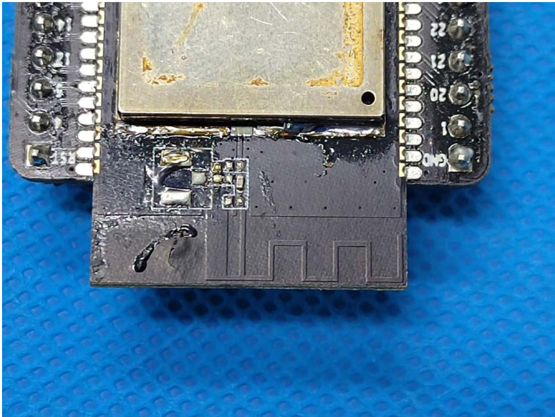
X-C13SL-1 Antenna
