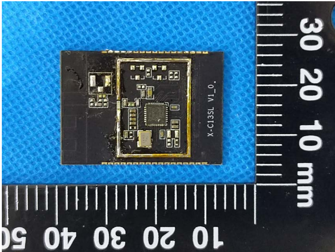
X-C13SL-1 Antenna
