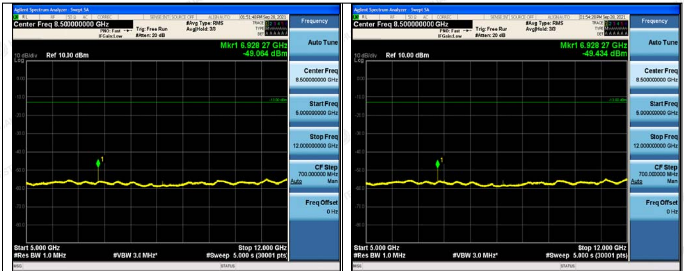
5GHz~12GHz
