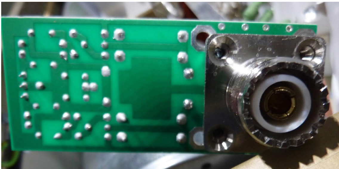
PCB – PWR meter V14
