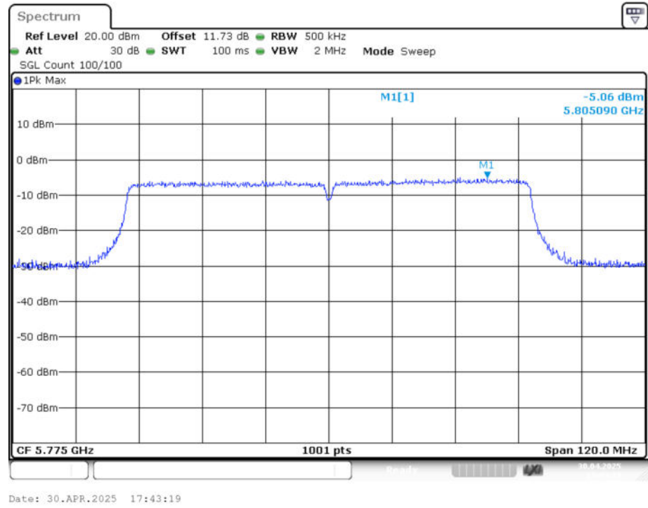
PSD NVNT ac80 5775MHz Ant1
