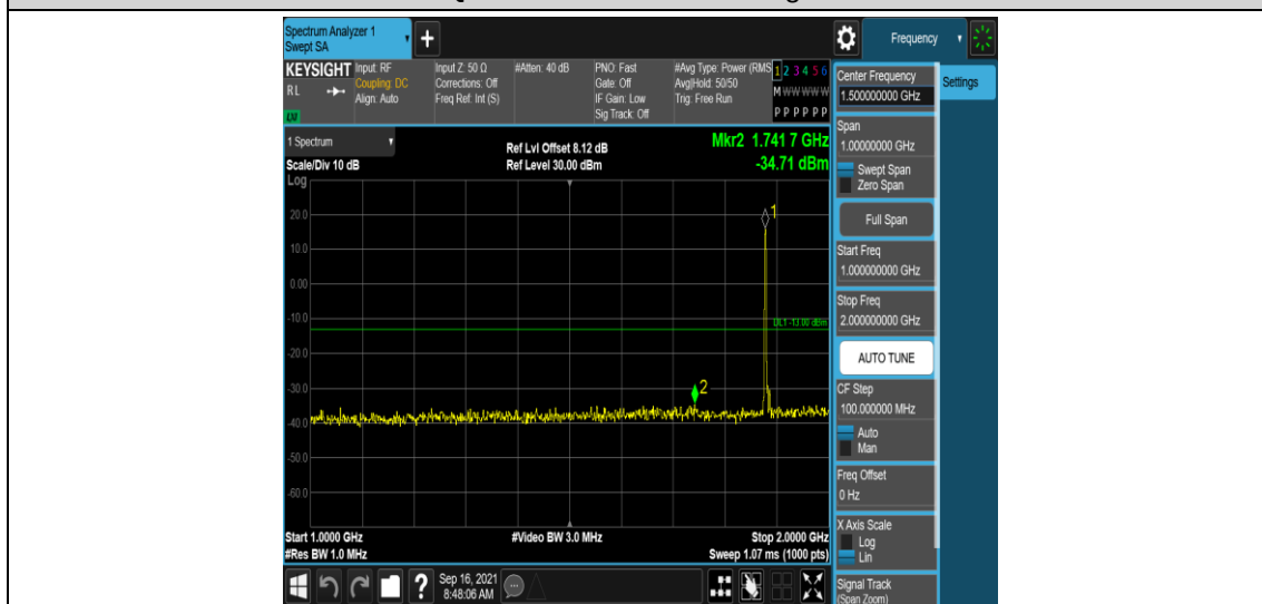
Band2-5MHz-QPSK-18900-1RB#0-Range4:1000~2000MHz
