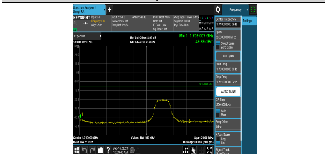
Band4-3MHz-QPSK-19965-1RB#14
