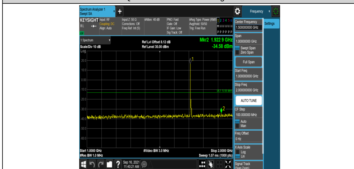
Band4-5MHz-QPSK-19975-1RB#0-Range4:1000~2000MHz
