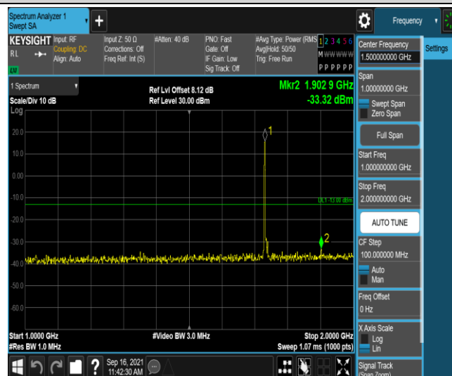
Band4-5MHz-QPSK-20175-1RB#0-Range4:1000~2000MHz
