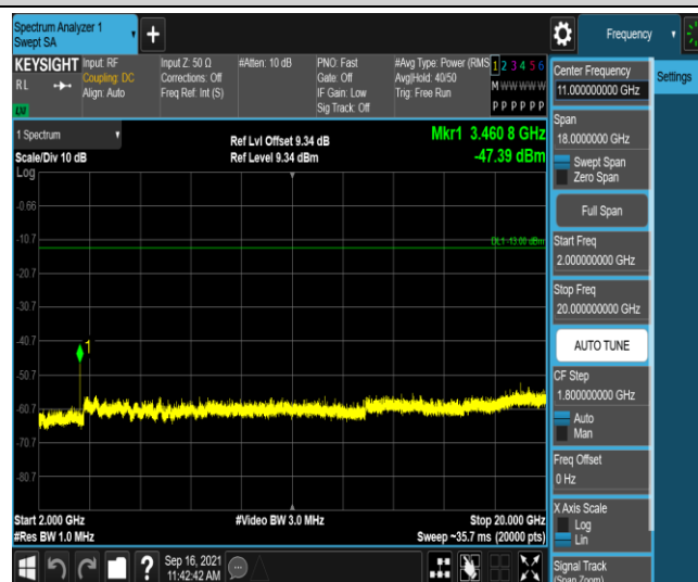
Band4-5MHz-QPSK-20175-1RB#0-Range5:2000~20000MHz
