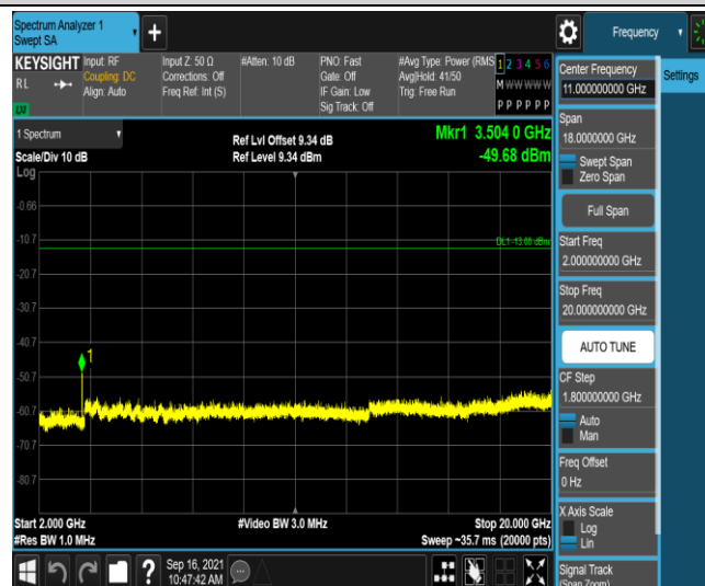
Band4-3MHz-QPSK-20385-1RB#0-Range5:2000~20000MHz
