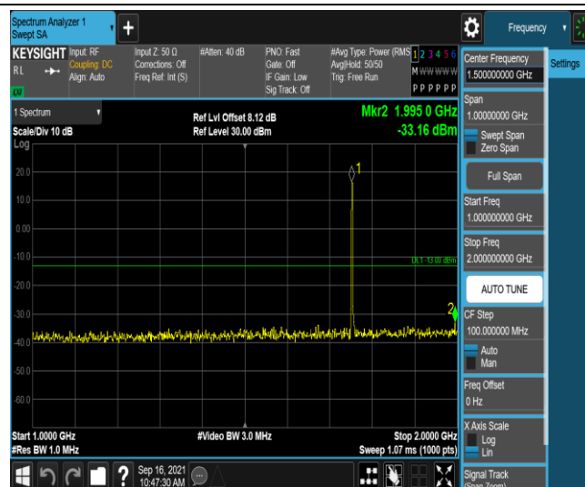
Band4-3MHz-QPSK-20385-1RB#0-Range4:1000~2000MHz
