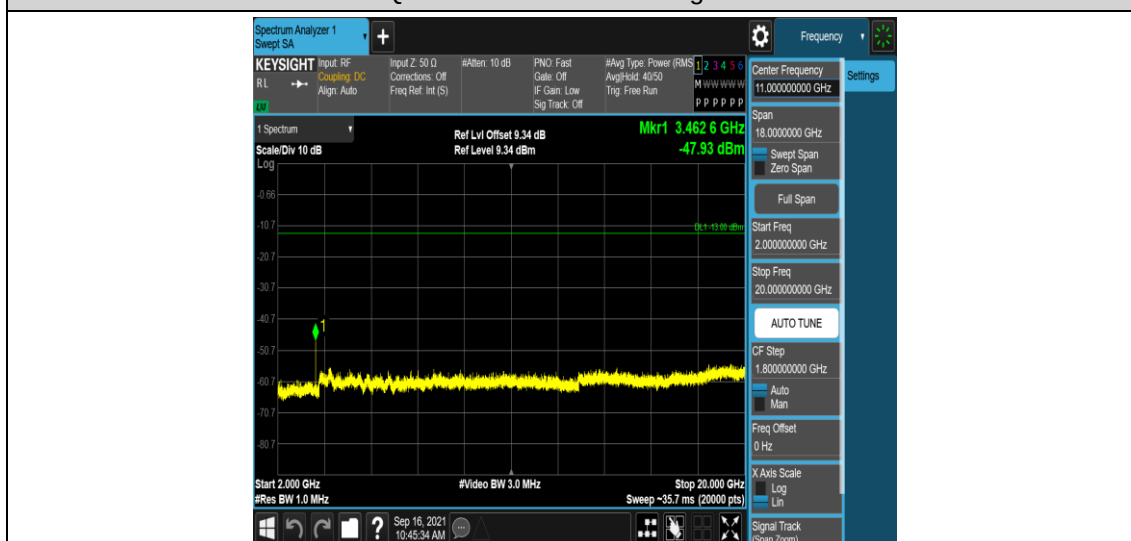
Band4-3MHz-QPSK-20175-1RB#0-Range5:2000~20000MHz
