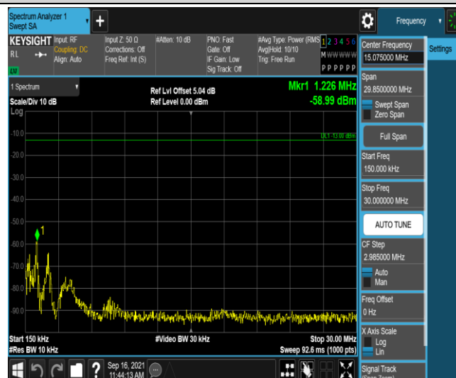
Band4-5MHz-QPSK-20375-1RB#0-Range2:0.15~30MHz
