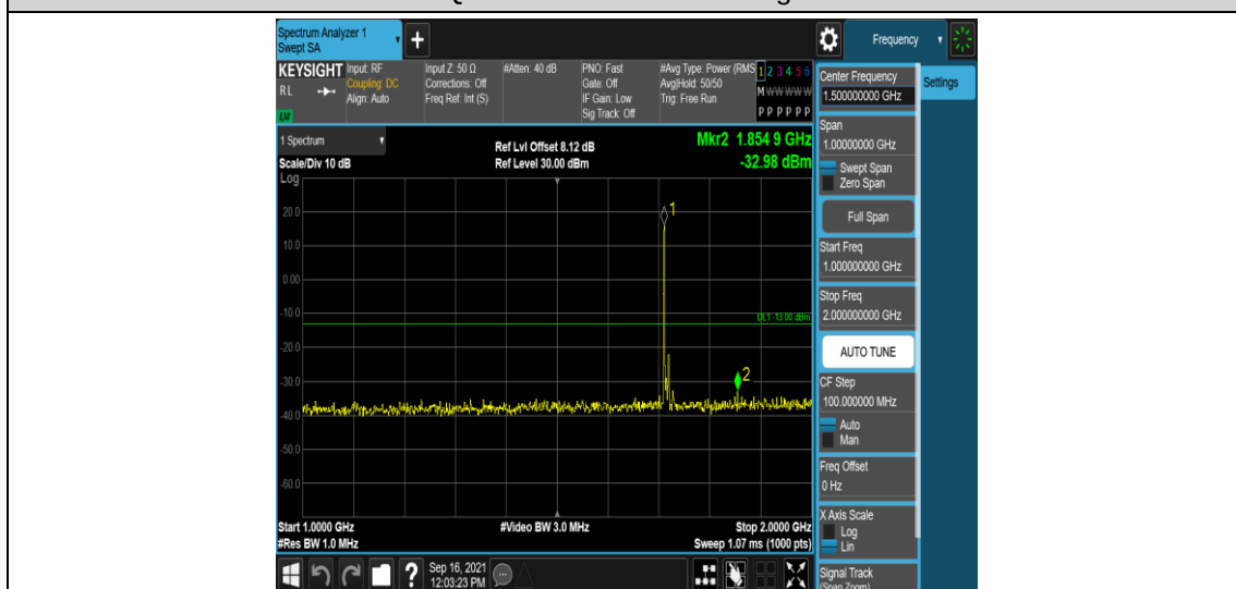
Band4-10MHz-QPSK-20000-1RB#0-Range4:1000~2000MHz
