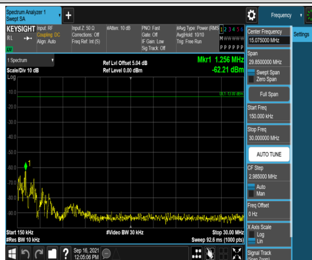
Band4-10MHz-QPSK-20175-1RB#0-Range2:0.15~30MHz
