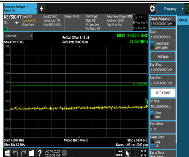
Band4-10MHz-QPSK-20175-1RB#0-Range4:1000~2000MHz
