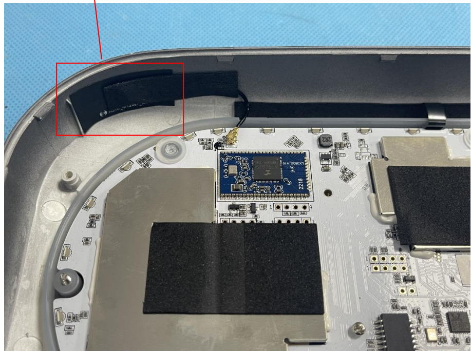
BT Ant.
