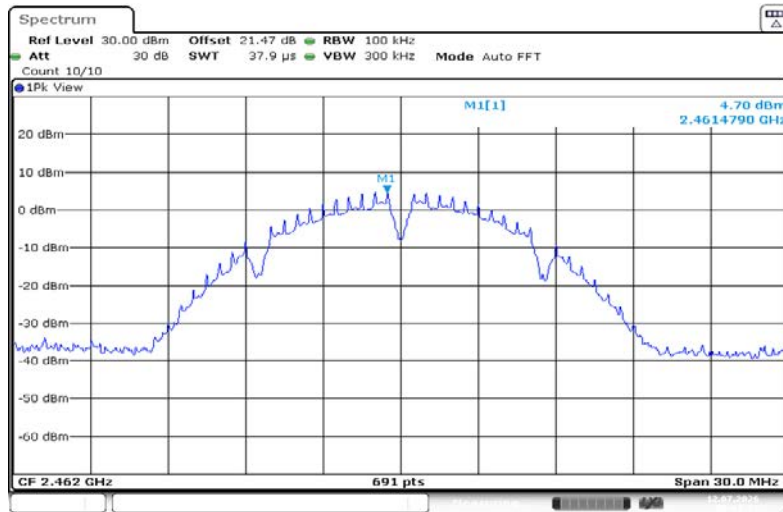
11B-Ant1-2462-0-Reference-PASS
