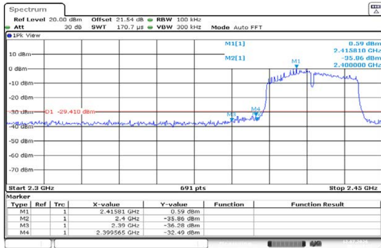
11N40ISO-Ant1-2422-PASS
