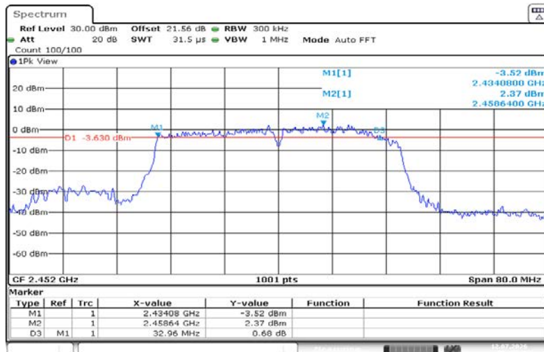
11N40ISO-Ant1-2452-PASS
