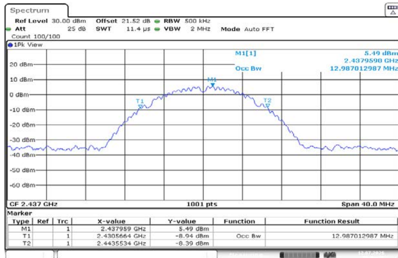
11B-Ant1-2437
