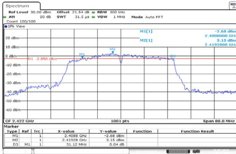
11N40ISO-Ant1-2422-PASS
