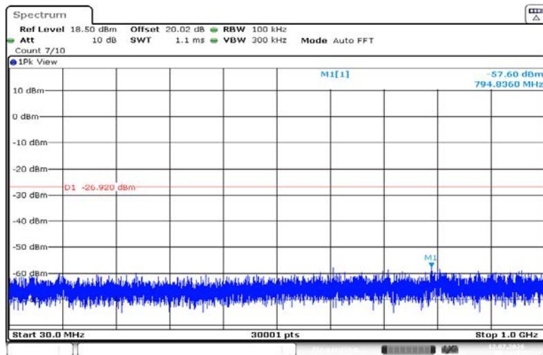
11G-Ant1-2437-30~1000-PASS
