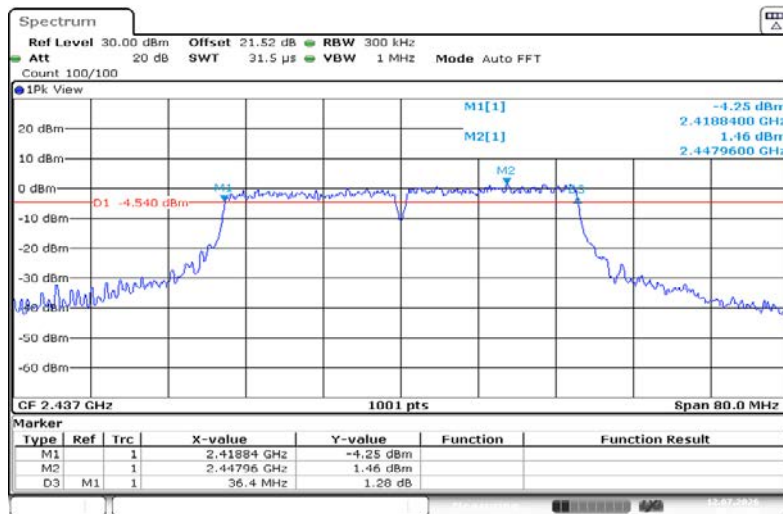
11N40ISO-Ant1-2437-PASS
