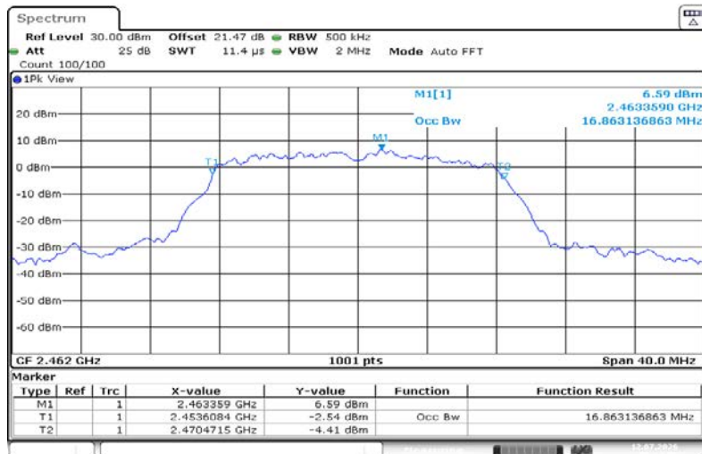
11G-Ant1-2462
