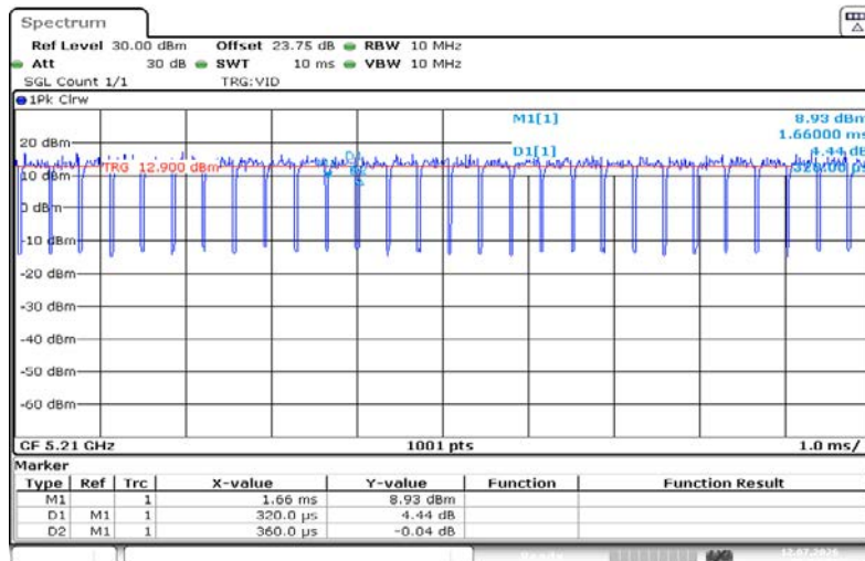
NTNV-11AC80SISO-Ant1-5210
