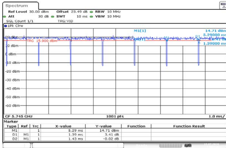
NTNV-11A-Ant1-5745
