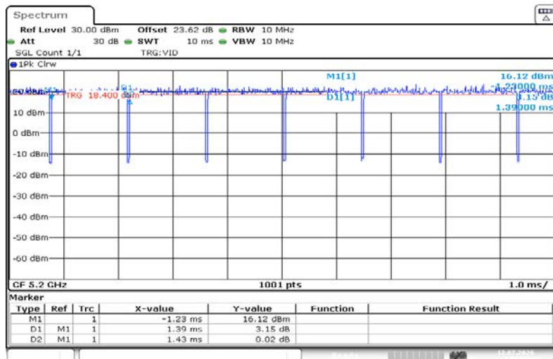
NTNV-11A-Ant1-5200
