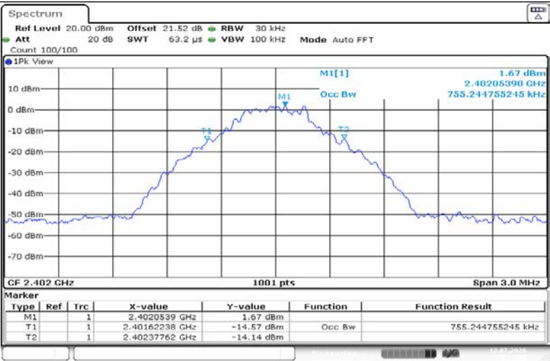
DH5-Ant1-2402
