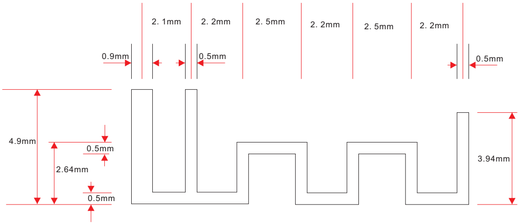
蓝牙天线尺寸图
