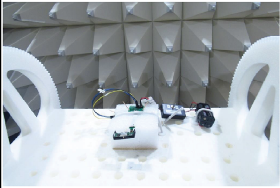
EUT Test Setup
