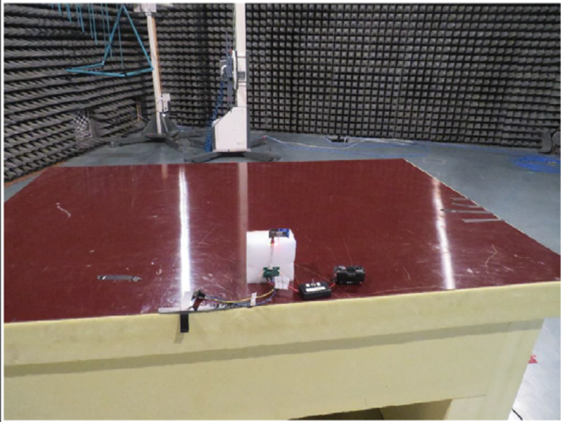
EUT Test Setup
