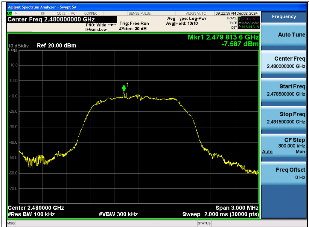
Test_Graph_EDR_ANT1_2480_3Mbps_Reference Level
