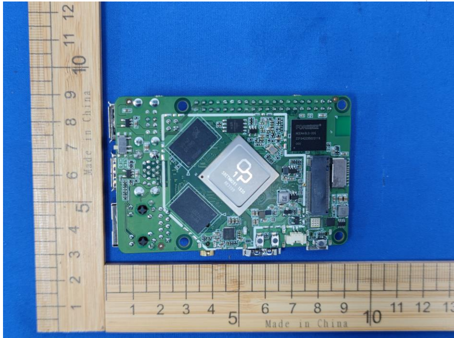
EUT Photo 2
