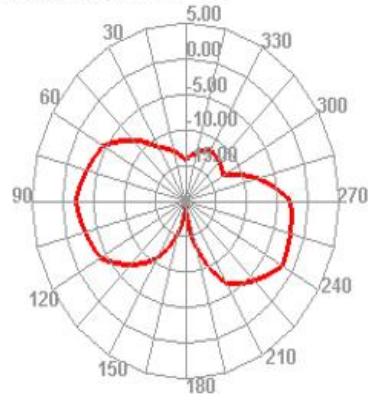
2400.000MHz E1
