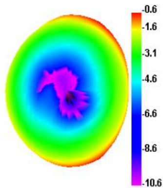
2400.000MHz E1
