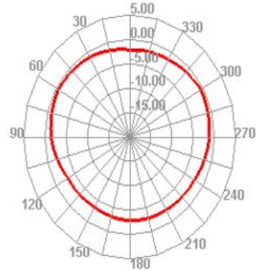
2400.000MHz E2
