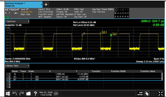
BLE 1M_Channel 19
