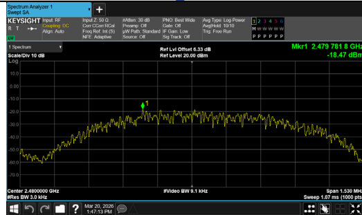
BLE 1M Channel 39
