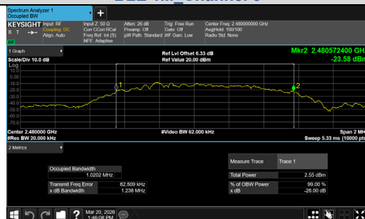
BLE 1M_Channel 39
