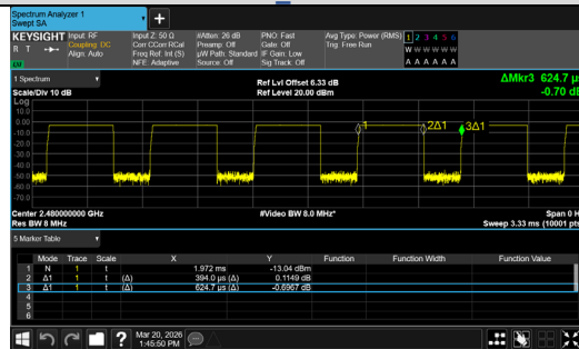
BLE 1M_Channel 39
