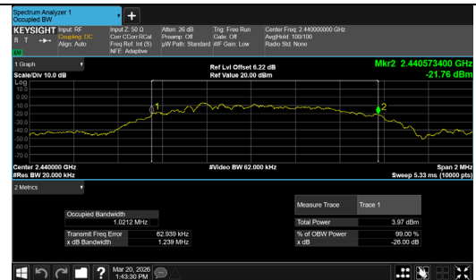
BLE 1M_Channel 19
