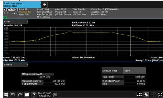
BLE 1M_Channel 0
