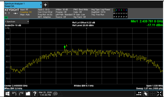
BLE 1M Channel 19
