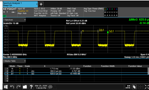
BLE 1M_Channel 0
