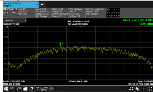
BLE 1M Channel 0
