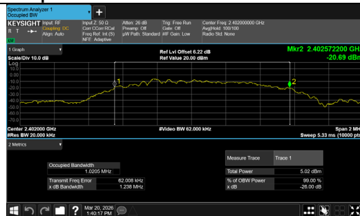
BLE 1M_Channel 0
