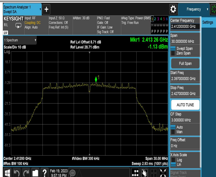
11N20CDD_Ant1_2412_0~Reference
