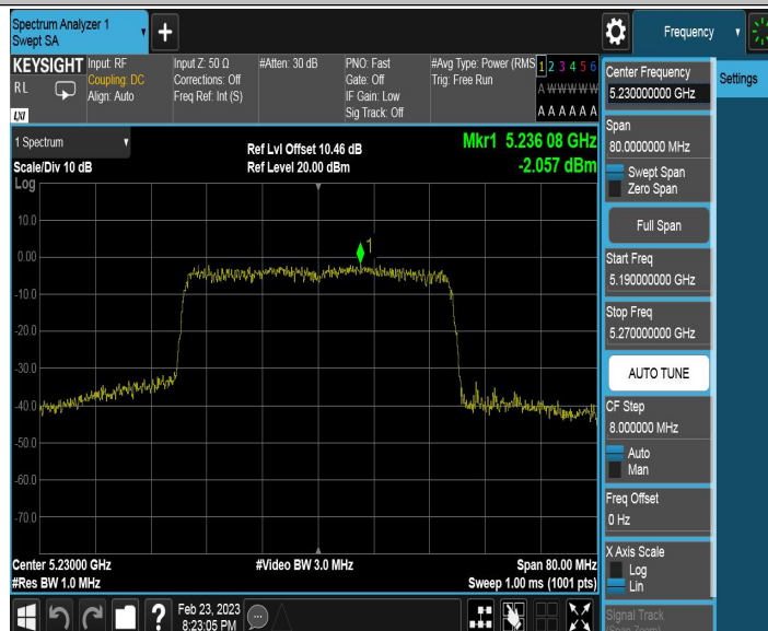
11AX40CDD_Ant2_5230
