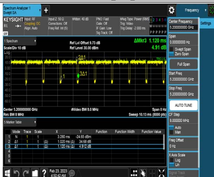
11AX20ISO_Ant2_5200
