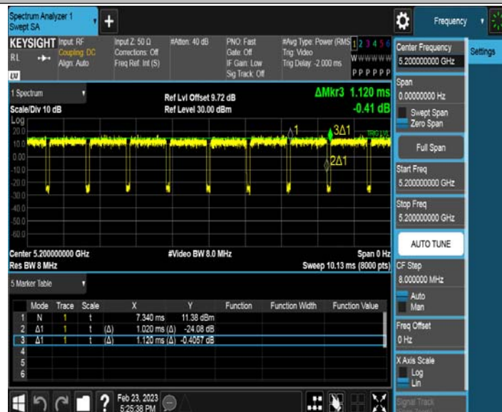
11AX20MIMO_Ant2_5200
