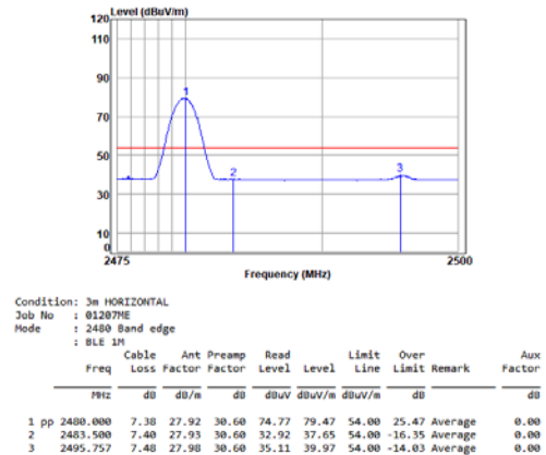
BLE_1M_TX_CH_39_Horizontal-AVG
