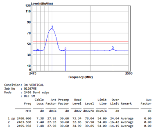
BLE_1M_TX_CH_39_Vertical-AVG
