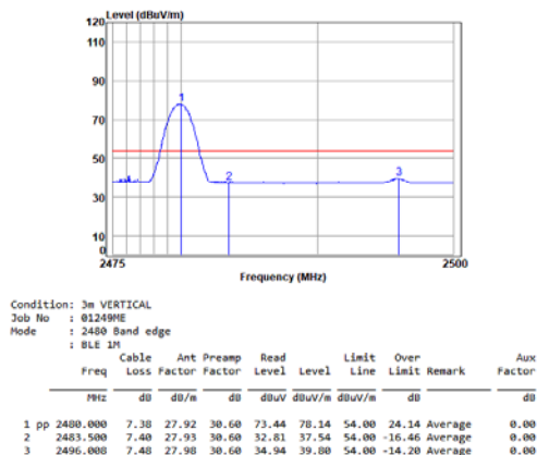
BLE_1M_TX_CH_39_Vertical-AVG
