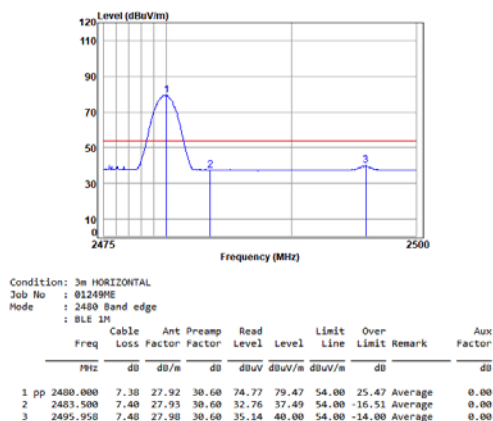
BLE_1M_TX_CH_39_Horizontal-AVG
