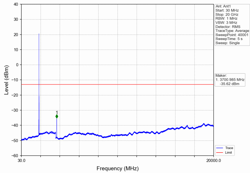
Band2_10MHz_16QAM_LCH_1855MHz_RB_50_0_NTNV
