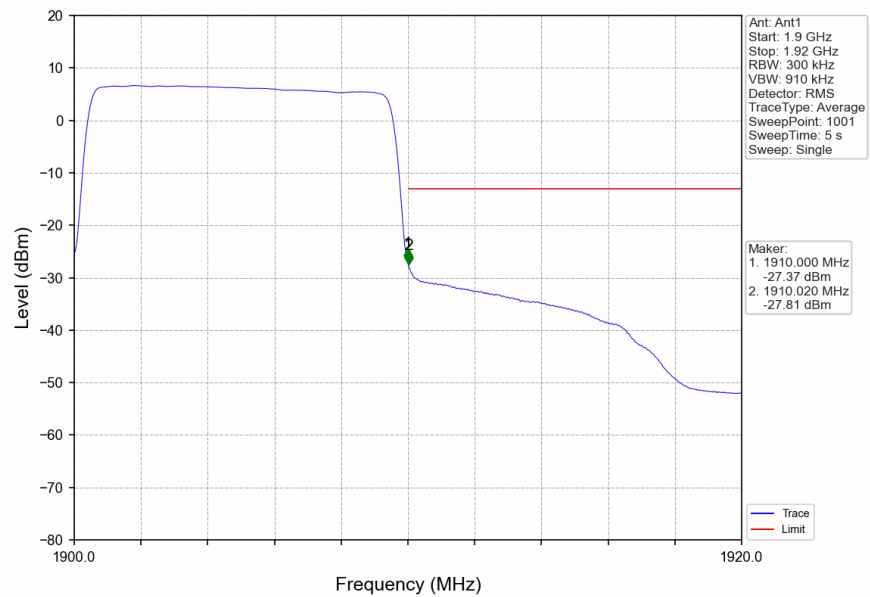
Band2_10MHz_16QAM_HCH_1905MHz_RB_50_0_NTNV
