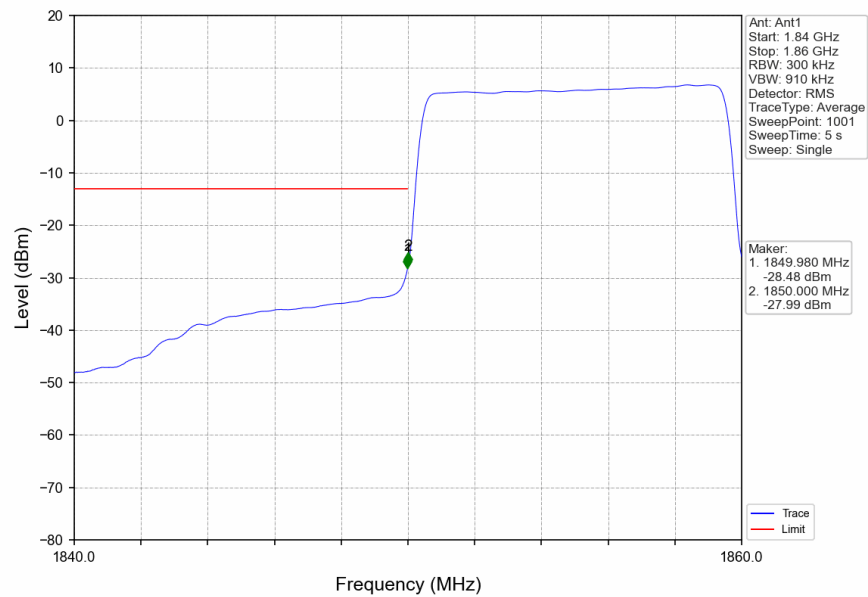
Band2_10MHz_16QAM_LCH_1855MHz_RB_50_0_NTNV
