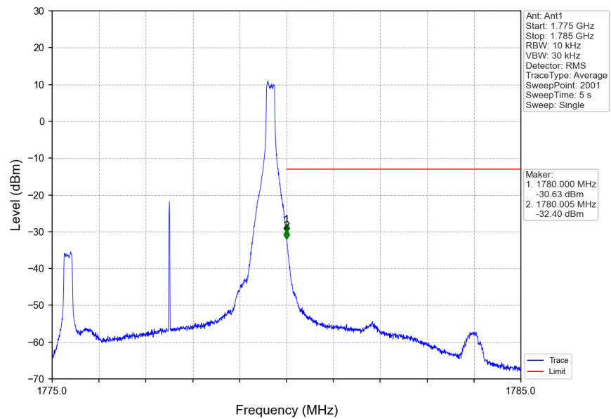
Band66_5MHz_QPSK_HCH_1777.5MHz_RB_1_24_NTNV
