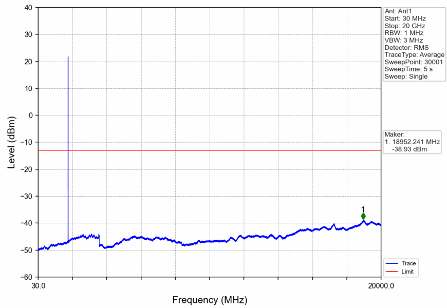
Band66_5MHz_QPSK_HCH_1777.5MHz_RB_1_24_NTNV
