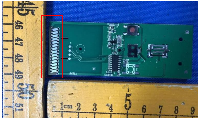
antenna
