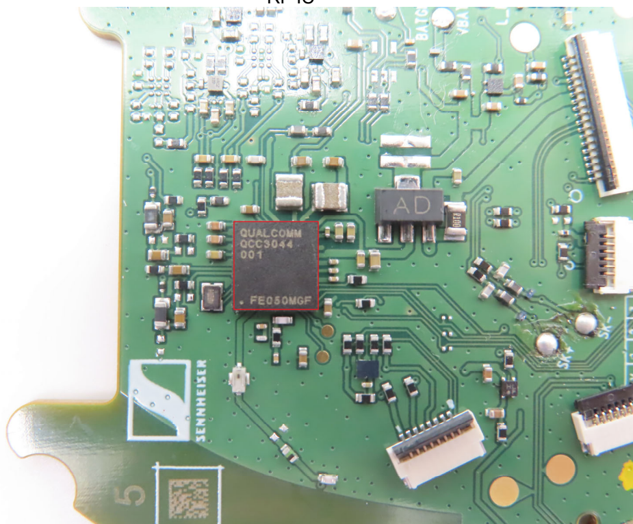
RF IC
