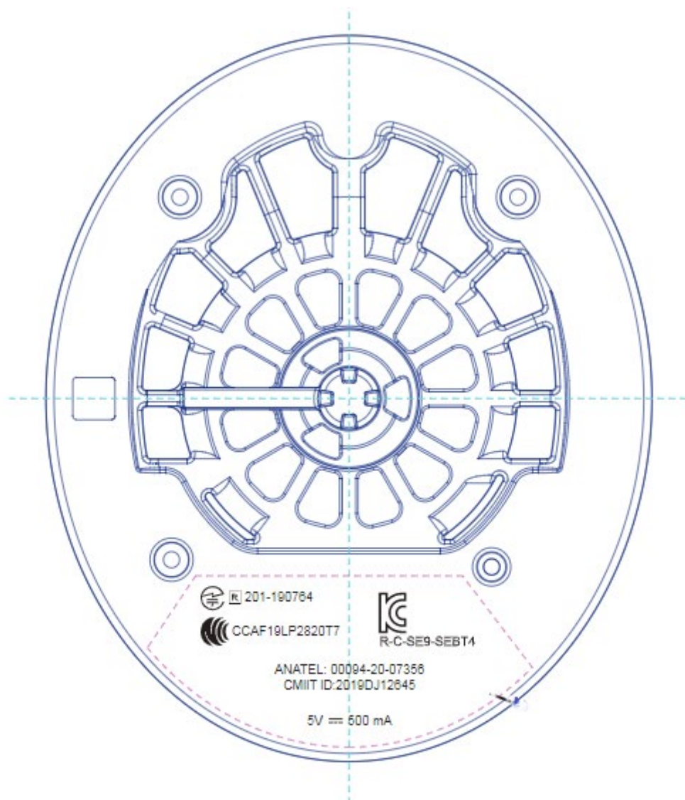
HD450BT Baffle plate R HD 450BT BLACK
