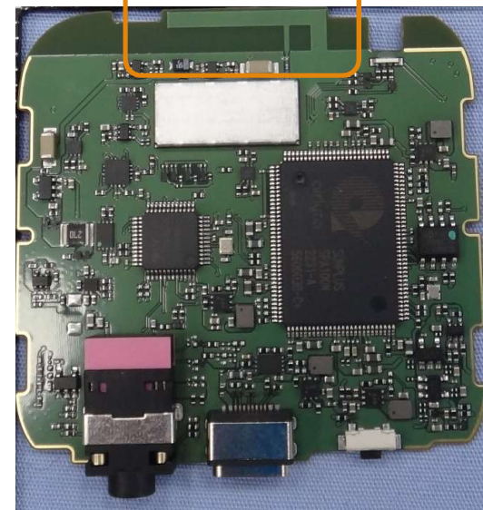
Antenna
