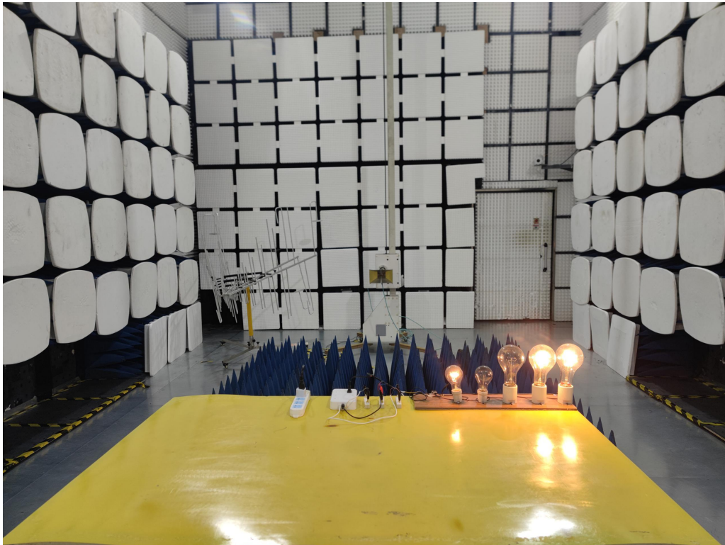
Fig. 2 (Above 1GHz)
