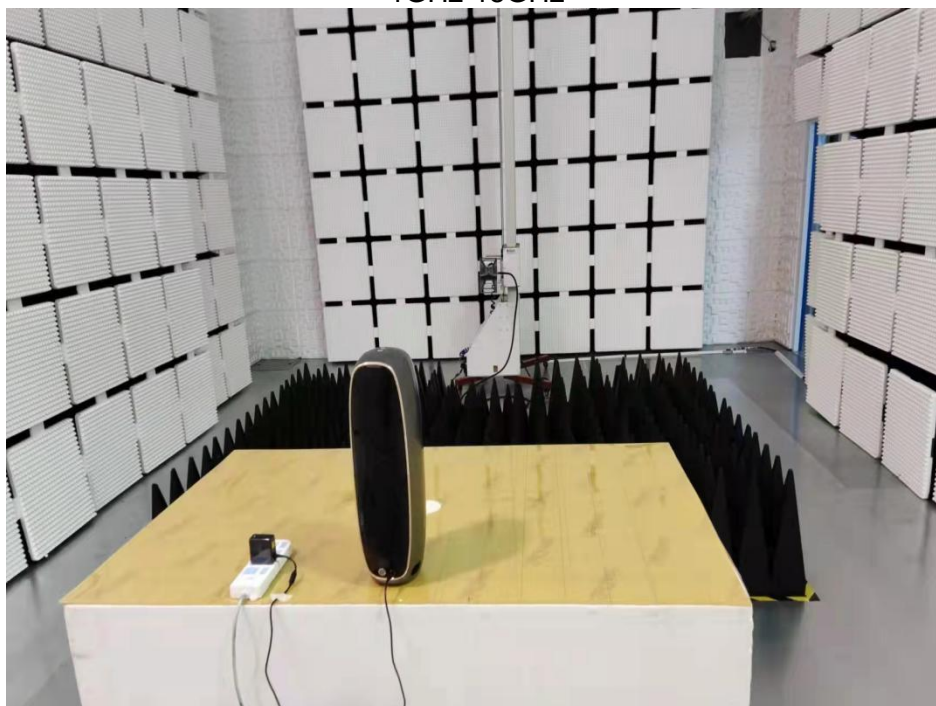
1GHz-18GHz
