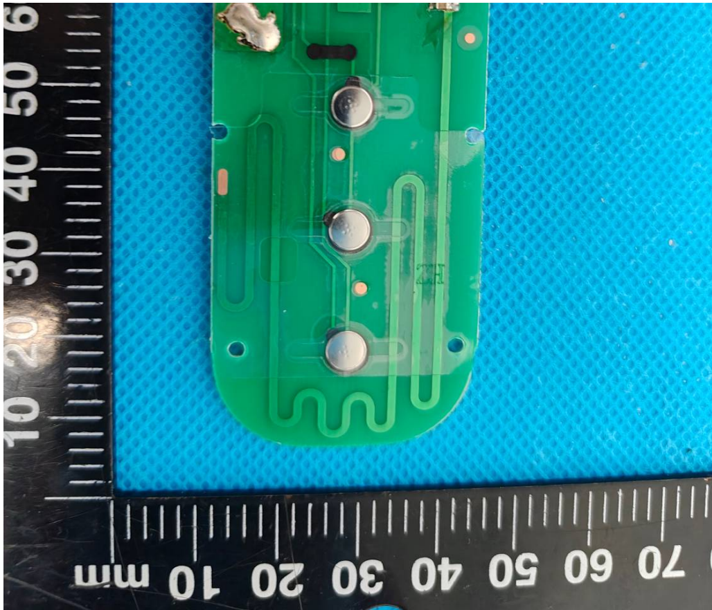
Antenna
