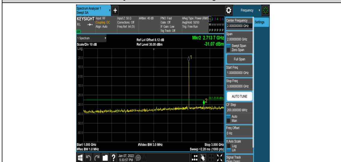
Band7-5MHz-QPSK-20775-1RB#0-Range4:1000~3000MHz
