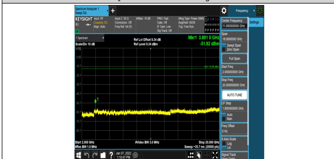
Band2-10MHz-QPSK-19150-1RB#0-Range5:2000~20000MHz
