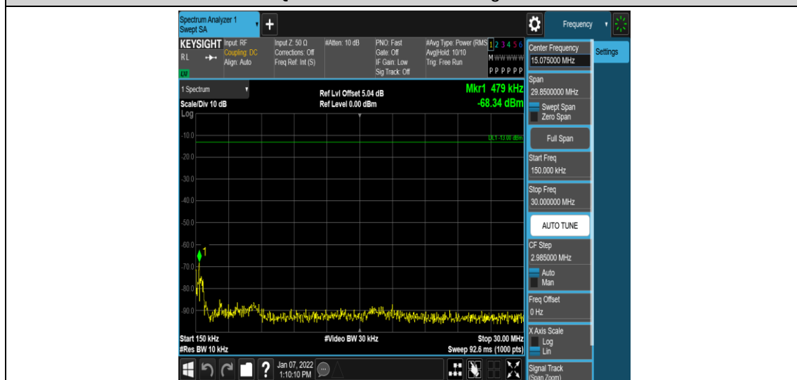
Band2-10MHz-QPSK-19150-1RB#0-Range2:0.15~30MHz
