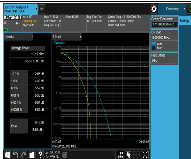
Band4-10MHz-QPSK-20000-1RB#0
