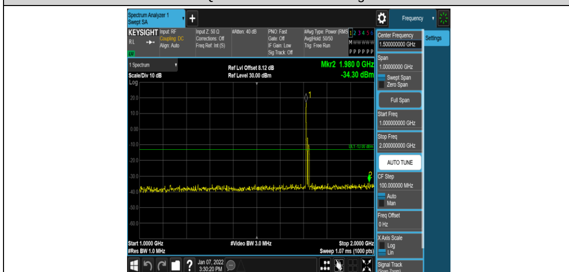
Band4-15MHz-QPSK-20025-1RB#0-Range4:1000~2000MHz
