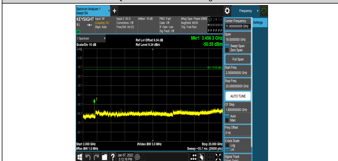
Band4-10MHz-QPSK-20175-1RB#0-Range5:2000~20000MHz
