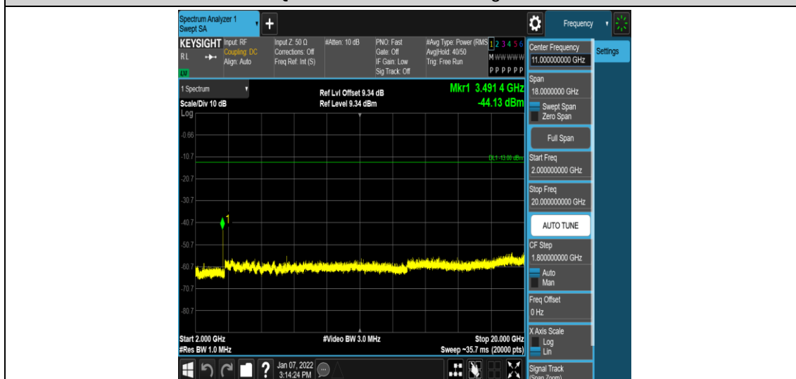
Band4-10MHz-QPSK-20350-1RB#0-Range5:2000~20000MHz
