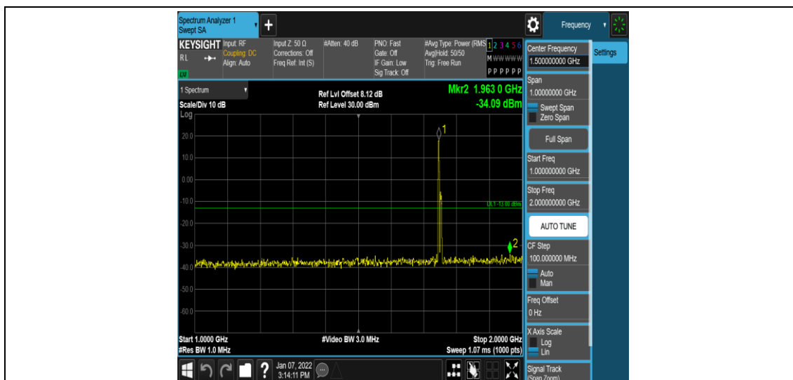
Band4-10MHz-QPSK-20350-1RB#0-Range4:1000~2000MHz
