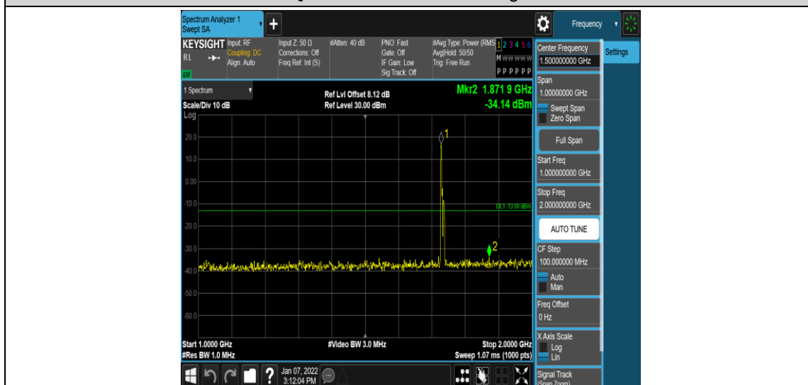
Band4-10MHz-QPSK-20175-1RB#0-Range4:1000~2000MHz
