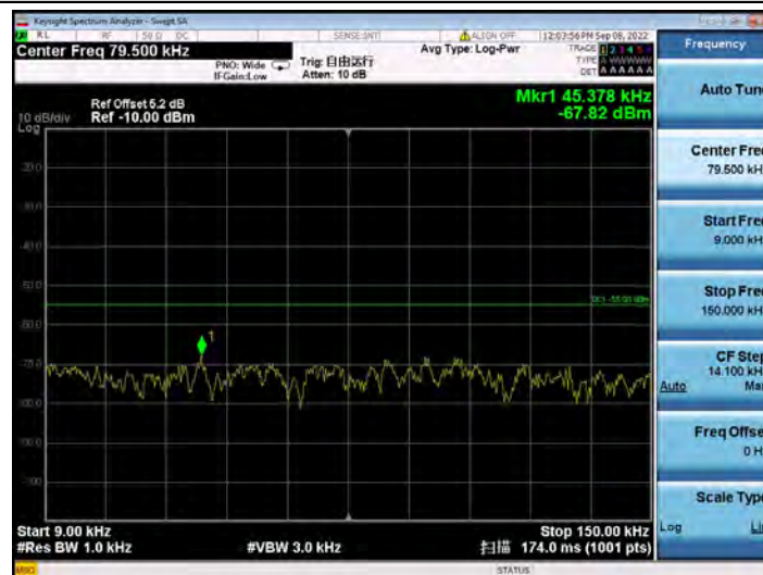
Band41-20MHz-QPSK-21100-1RB#0-Range1:9KHz~150KHz
