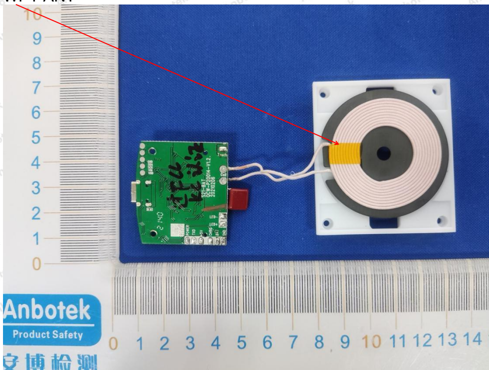
WPT ANT
