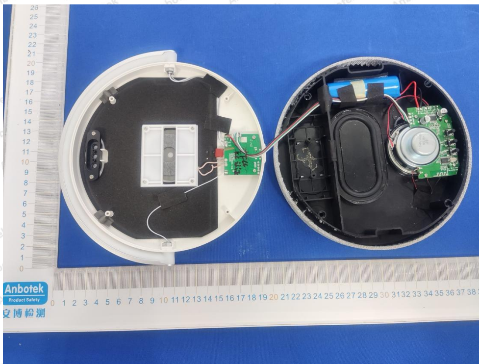
WPT ANT
