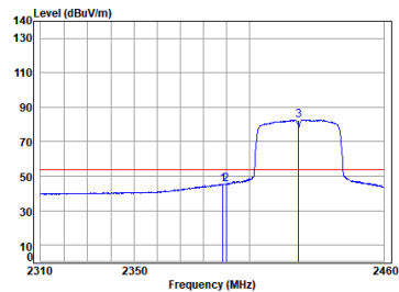
11n_HT(40M)_TX_CH_03_Vertical-Avg
