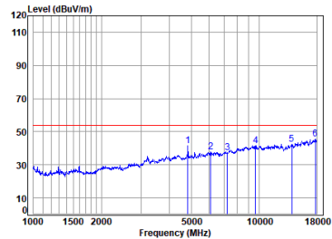
11n_HT(20M)_TX_CH_01_Vertical-Avg
