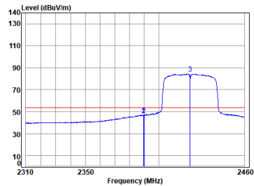
11n_HT(40M)_TX_CH_03_Horizontal-Avg
