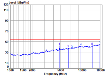
11n_HT(20M)_TX_CH_01_Horizontal-Avg
