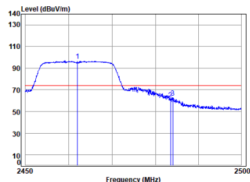
11n_HT(20M)_TX_CH_11_Horizontal-Peak
