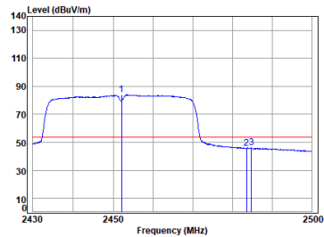
11n_HT(40M)_TX_CH_09_Horizontal-Avg
