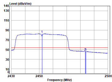
11n_HT(40M)_TX_CH_09_Vertical-Avg
