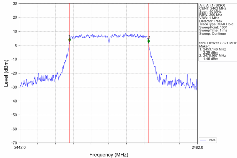
802.11n(HT20)_HCH_2462MHz_Ant1 (SISO)_NTNV
