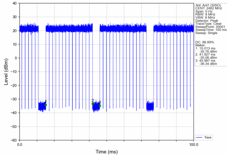
802.11n(HT20)_HCH_2462MHz_Ant1 (SISO)_NTNV
